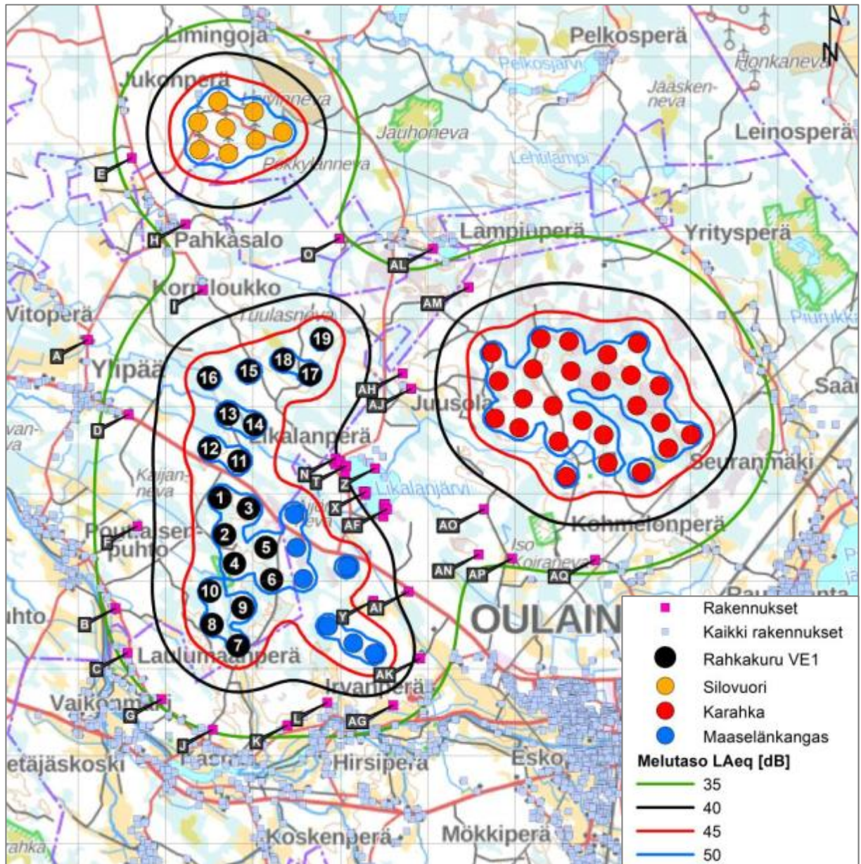
Kuva 35. Rahkakurun tuulipuiston melumallinnus VE1 -suunnitelma. (Lähde: Rahkakurun tuulivoimapuisto, Merijärvi, Suomi: Melu- ja väkelaskelmat. Kjeller Vindteknikk Oy, 2024)
