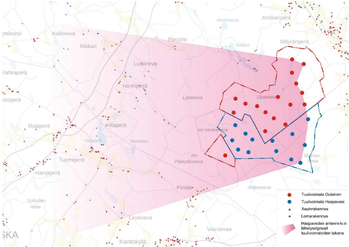
Kuva 31 Rahkola-Hautakankaan tuulivoimalat voivat häiritä antenni- tv –vastaanottoa alueella, jossa tuulivoimalat sijoittuvat Haapaveden lähetasemalta tulevan signaalin ja tv-vastaanottimen väliin.
