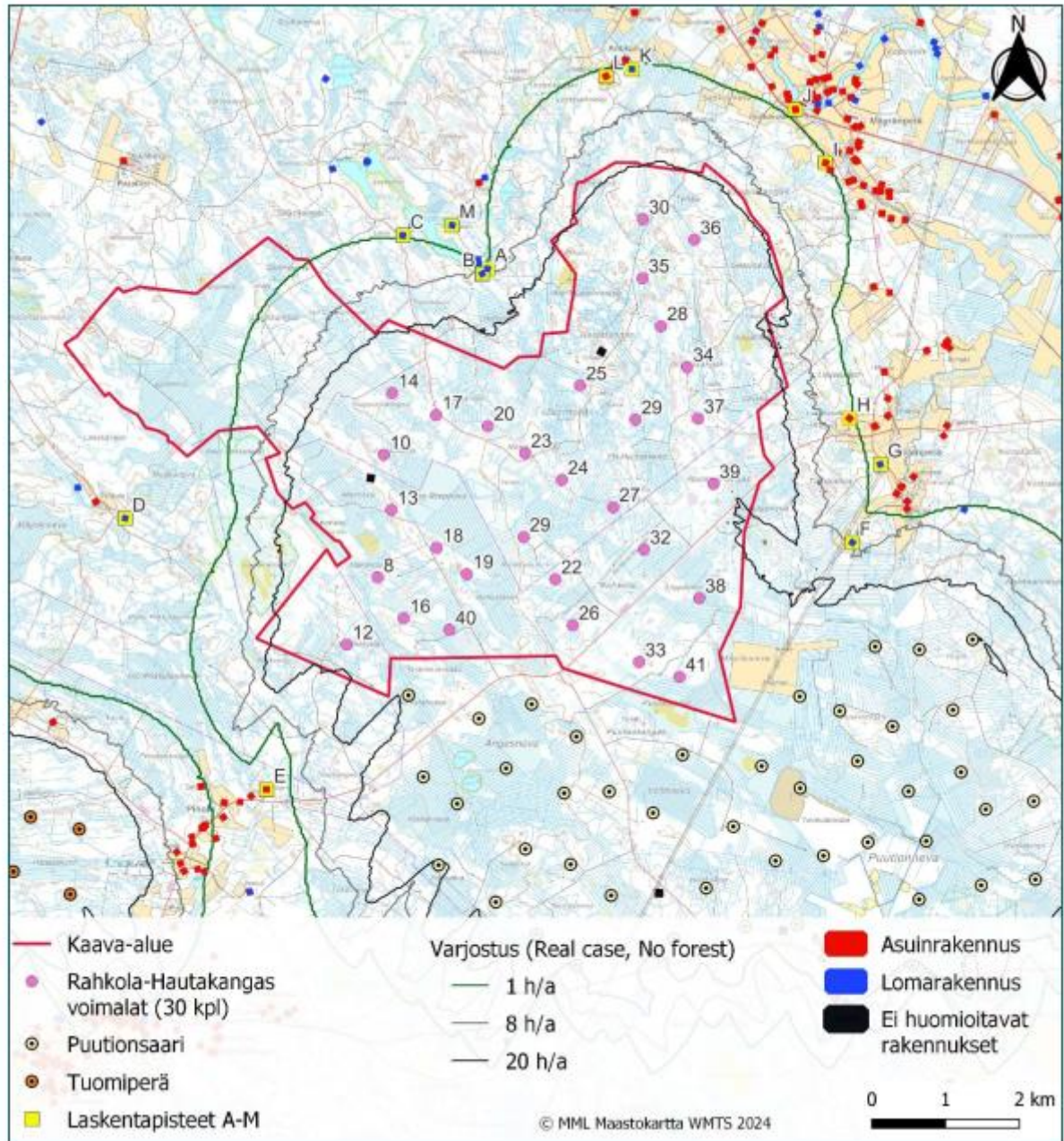
Kuva 28 Varjostusmallinnuksen tulos hankkeen toteutuessa, kun puuston suojaavaa vaikutusta ei ole huomioitu
