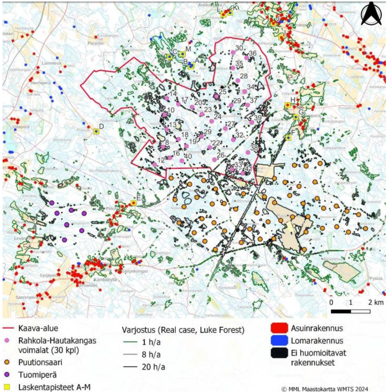
Kuva 29 Varjostusmallinnuksen tulos hankkeen toteutuessa, kun puuston suojaava vaikutus on huomioitu.
